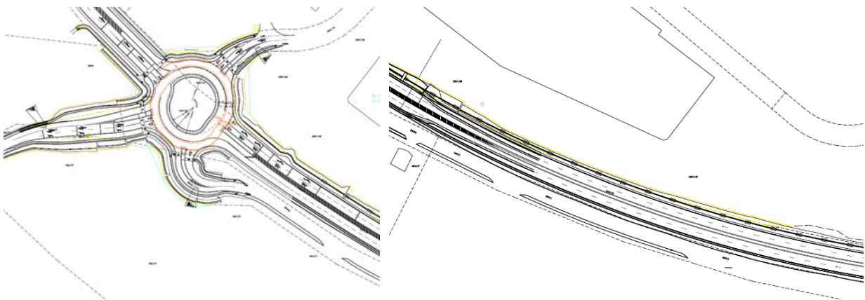
A turbókörforgalom és a hozzá kapcsolódó sávbővítés területi igényei (Forrás: NIF Zrt. - 2021.10.20.)
